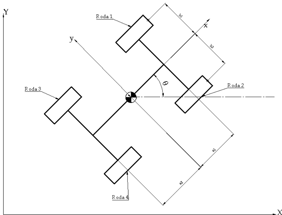
Figura 3.11- Veículo em movimento plano.
