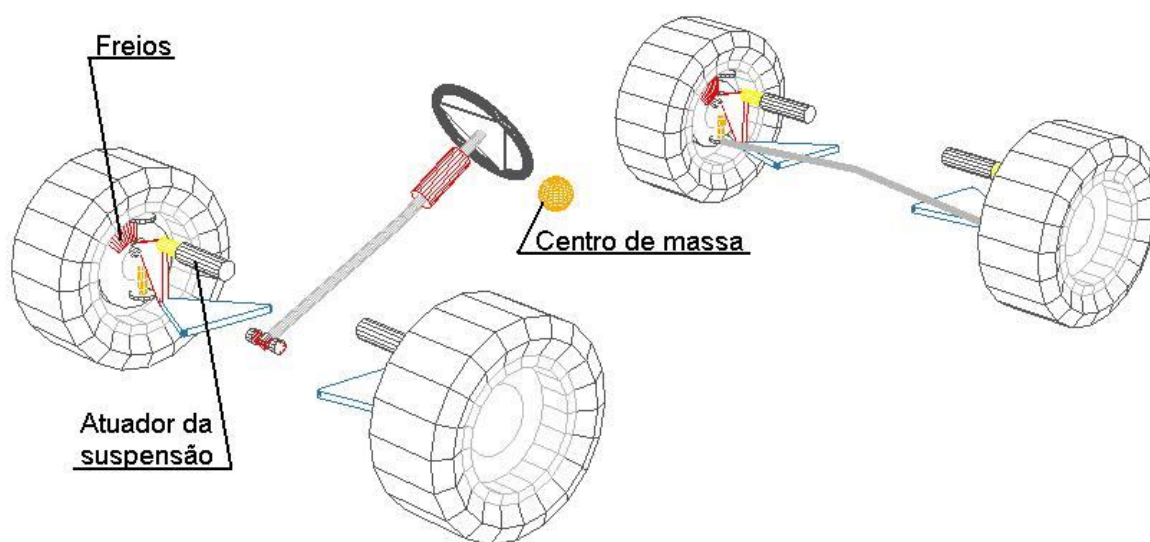
Figura 5.1 – Protótipo virtual no Adams/Car.
