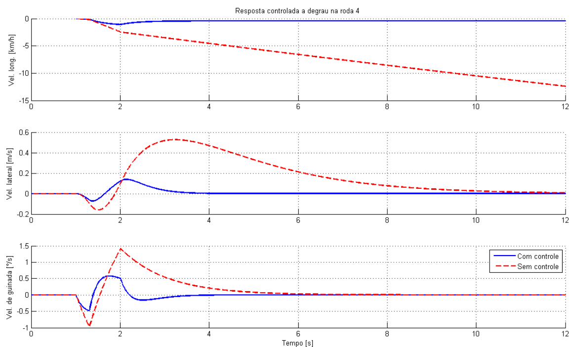
Figura 4.6 – Resposta do sistema com e sem controle para frenagem de emergência
