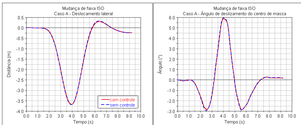
Figura 5.6 – Caso A com e sem controle de frenagem.
