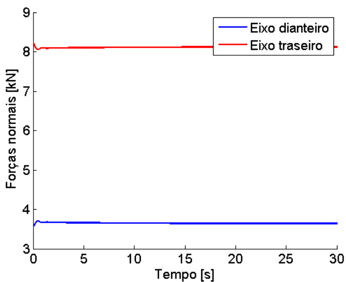
Figura 3.9 – Comportamento das forças normais nos eixos em função do tempo.
