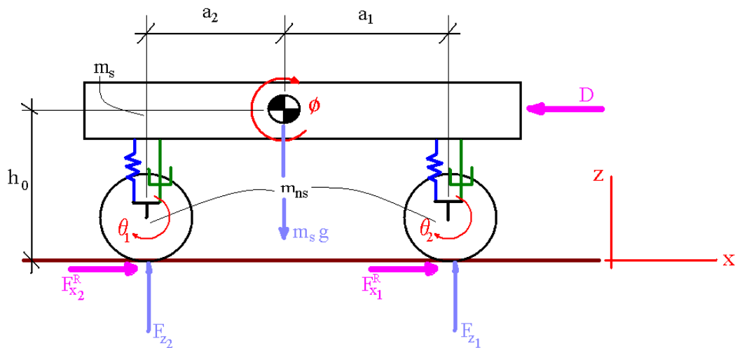
Figura 3.3 - Modelo de dinâmica longitudinal com 5 graus de liberdade.
