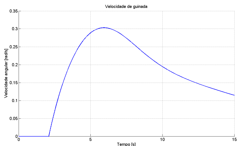
Figura 3.14 - Velocidade de guinada no modelo não linear.
