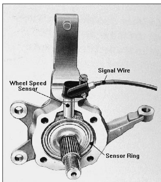
Figura 4.3 – Detalhe de manga de eixo mostrado o disco dentado e o sensor de velocidade.
