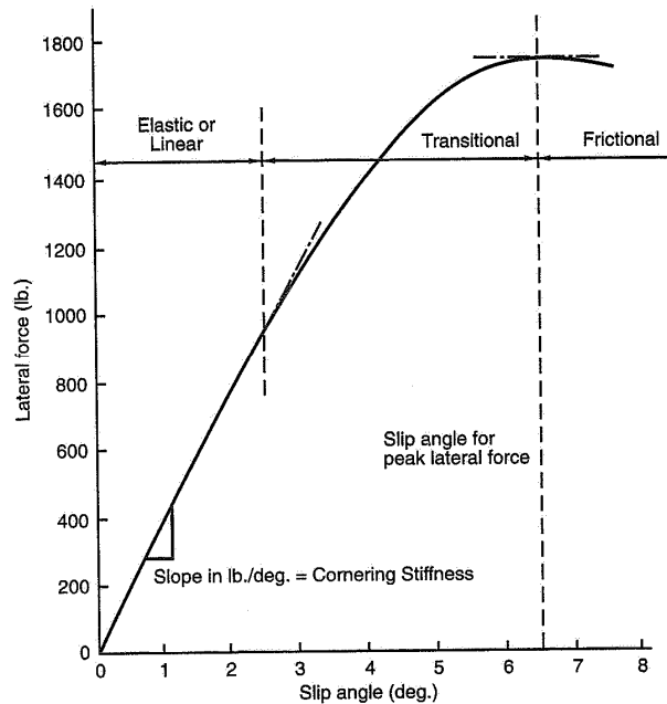
Figura 2.3 – Diagrama de força lateral ( F_y ) em função do escorregamento ( \alpha ), mostrando as fases de contato.
