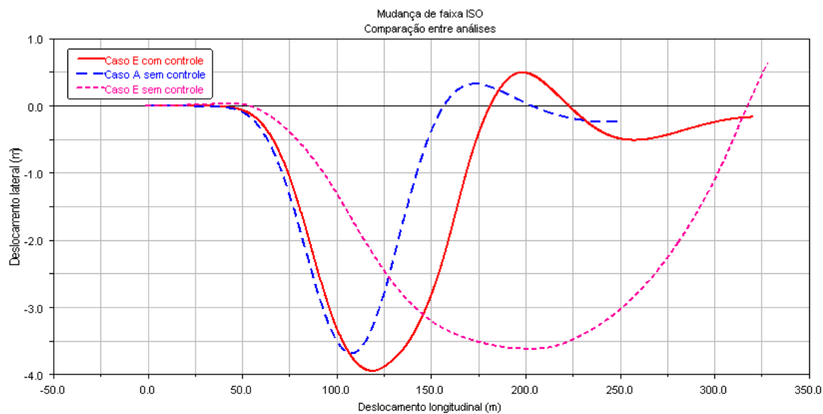
Figura 5.7 – Comparação entre simulação dos casos A e E sem controle e E com controle.
