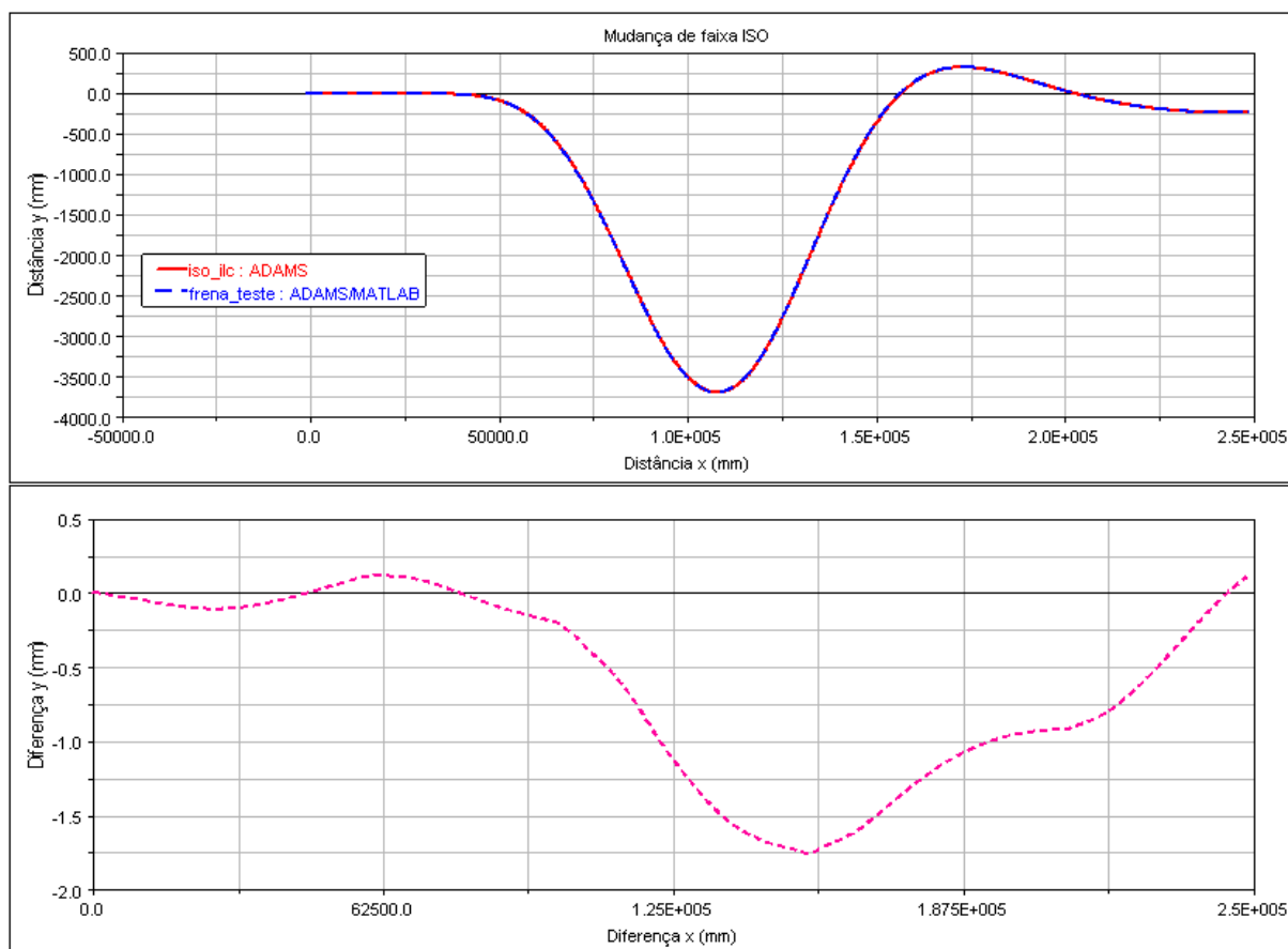
Figura 5.2 - Comparação entre duas simulações sem controle rodadas somente no Adams e com simulação paralela Matlab/Adams.
