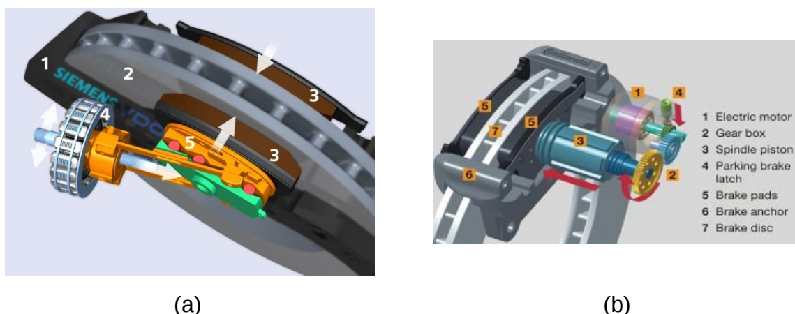
Figura 1.1 – Pinças de freios (a) EWB e (b) EMB.
