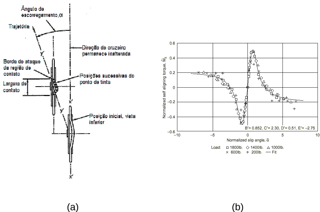
Figura 2.5 – (a) Roda em movimento não simétrico (adaptado de Milliken (1995)) e (b) curva típica de torque auto-alinhante ajustado pelo modelo MF de Pacejka (adaptado de MRA).
