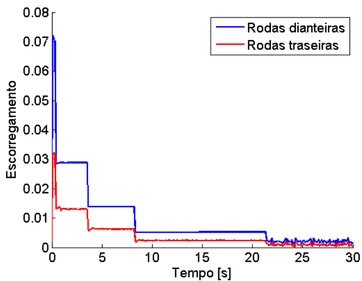
Figura 3.10 – Escorregamento longitudinal dos pneus em função do tempo.
