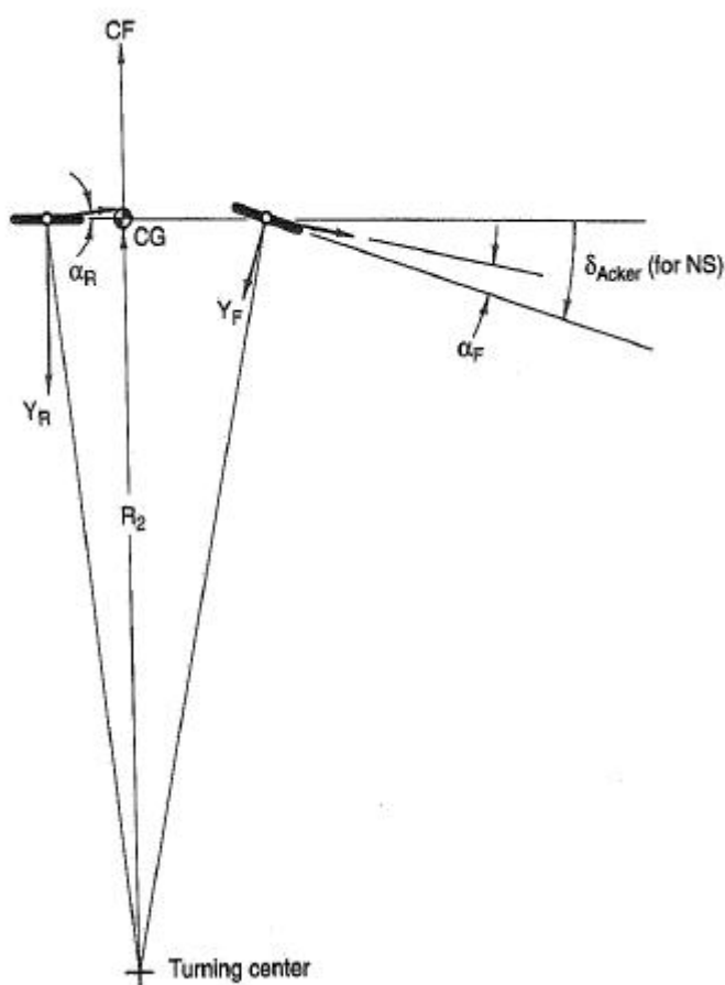
Figura 2.8 – Modelo de bicicleta para veículo executando curva.
