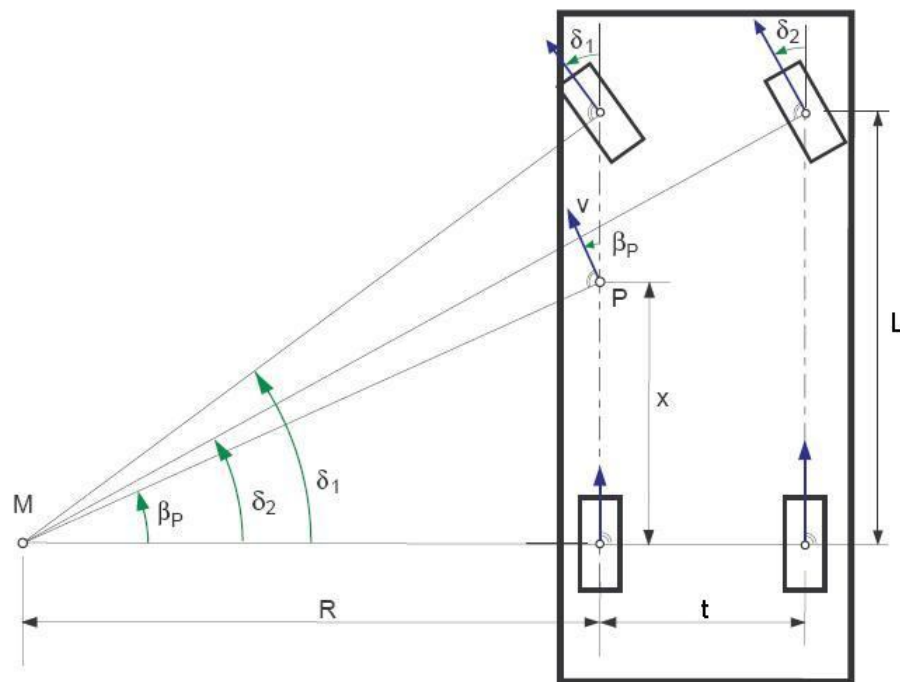
Figura 2.7 – Modelo de Ackerman (adaptado de Rill, 2007a).
