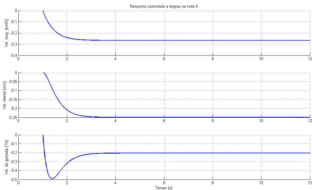
Figura 4.5: Resposta controlada ao degrau na roda traseira direita.
