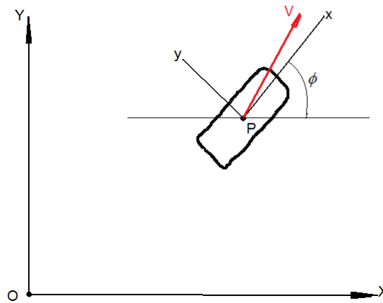
Figura 3.1 – Esquema para o estudo da dinâmica do pneu.
