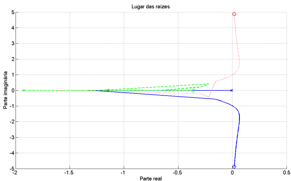
Figura 4.2 – Mapa do lugar das raízes para diversas combinações de condições iniciais.
