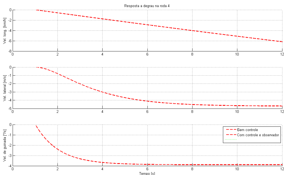
Figura 4.4: Resposta do sistema linearizado a entrada degrau na roda traseira direita.
