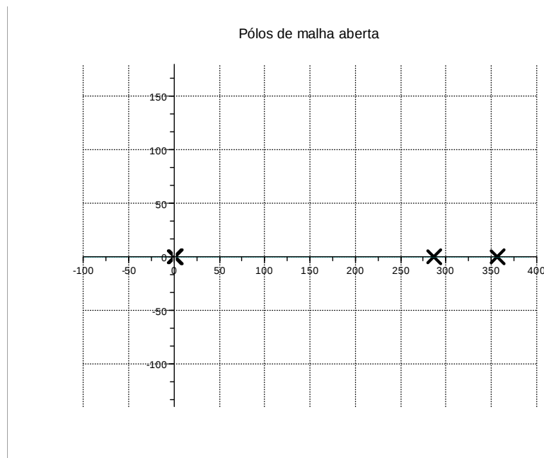
Figura 3.2 – Pólos de malha aberta do sistema
