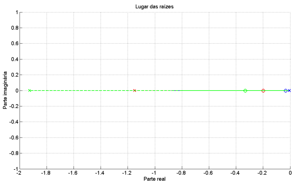
Figura 4.1 – Mapa do lugar das raízes para velocidade longitudinal entre 10 m/s (x) e 60 m/s (o).
