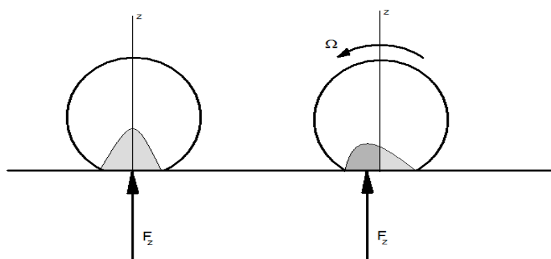
Figura 2.4 – Deslocamento da força vertical.
