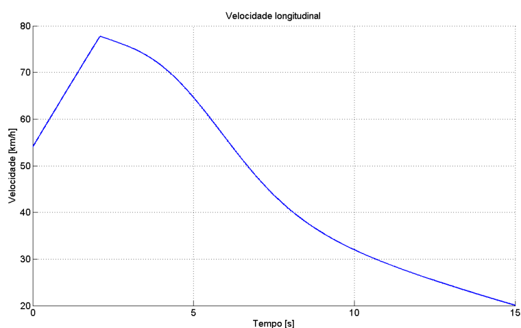
Figura 3.12 - Velocidade longitudinal no modelo não linear.
