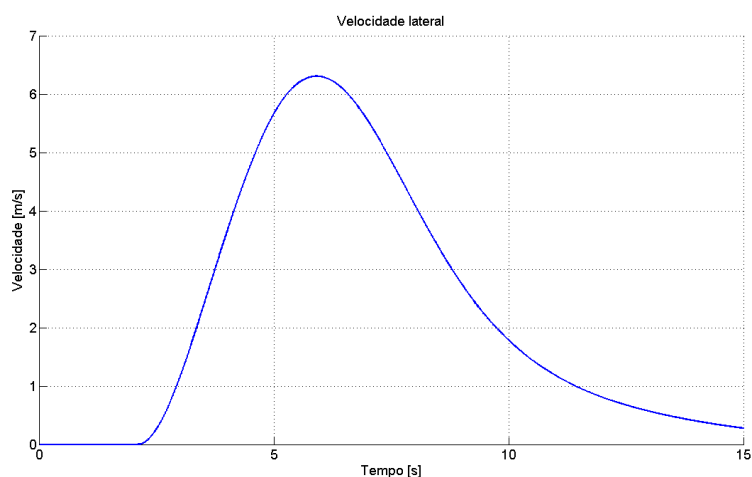
Figura 3.13 - Velocidade lateral no modelo não linear.
