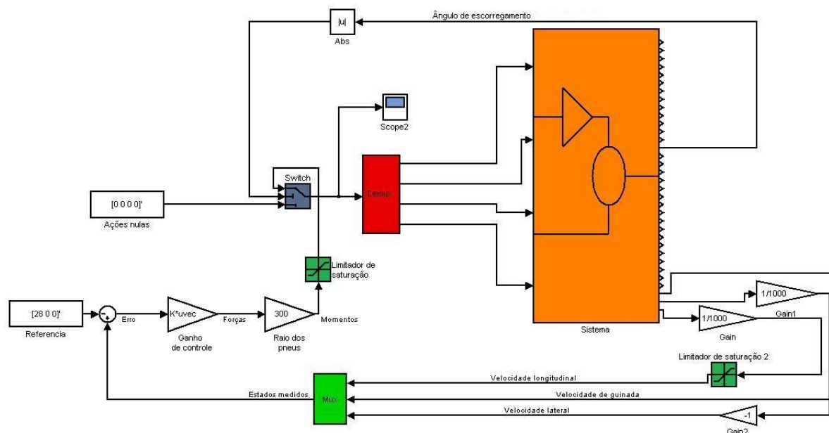
Figura 5.3 – Diagrama de blocos montado no Simulink.
