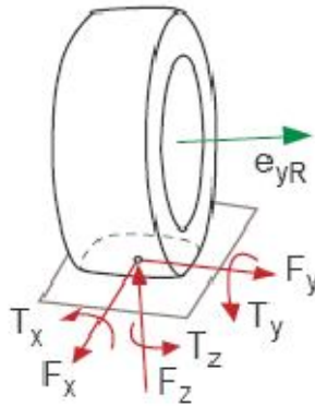
Figura 2.2 – Forças e momentos agindo sobre o pneu (adaptado de Rill ,2007).
