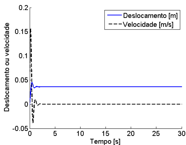
Figura 3.6 – Comportamento vertical em função do tempo.
