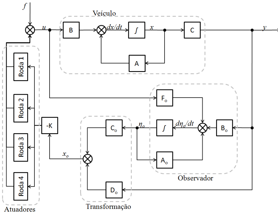
Figura 4.7 – Diagrama de blocos do sistema com controlador-observador.
