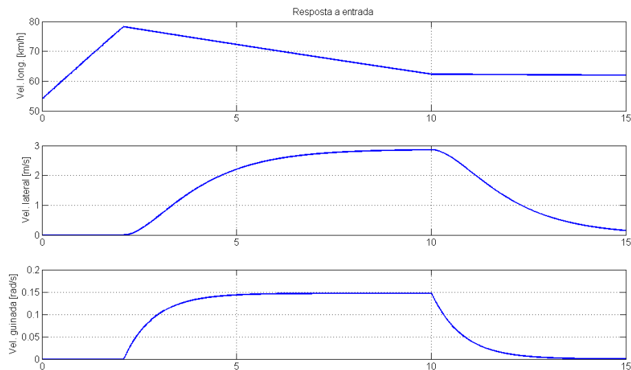
Figura 3.16 - Respostas do modelo linearizado.
