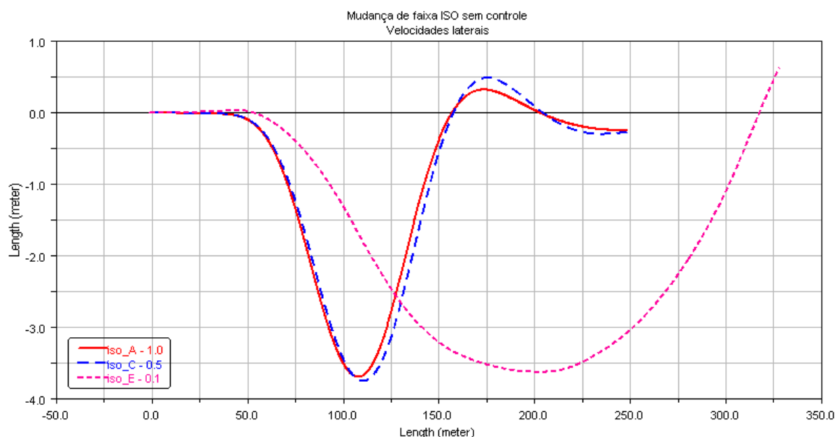
Figura 5.4 – Trajetória do veículo para três casos de pista sem controle nos freios.
